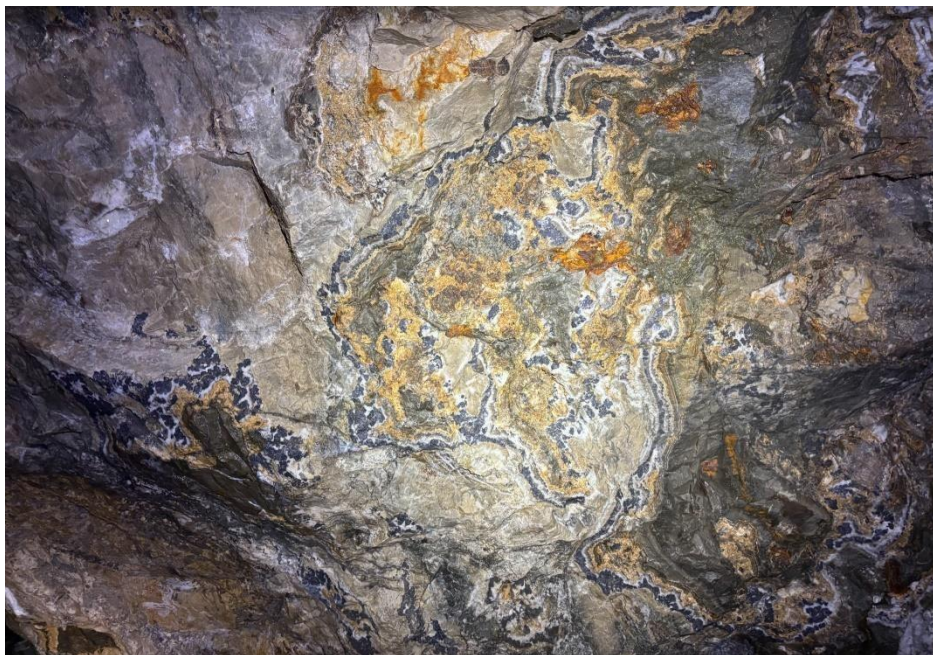
Kaotikus elhelyezkedésű galenit és szfalerit tartalmú erek.
